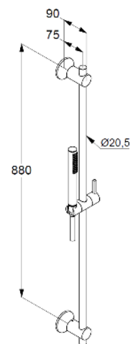
Maßzeichnung
