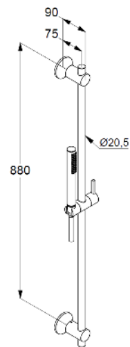
Maßzeichnung
