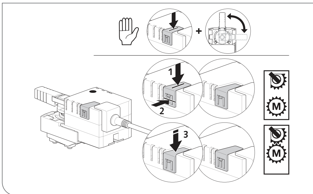
Abb 12: Handbetrieb (< DN 50)
