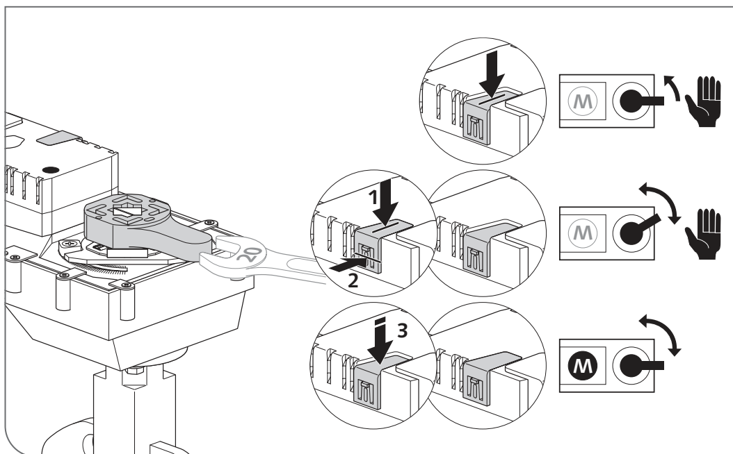
Abb 13: Handbetrieb (= DN 50)
