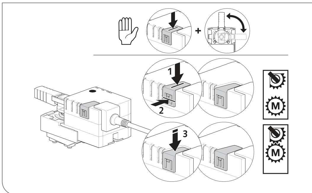
Abb 25: Manual mode (<DN 50)
