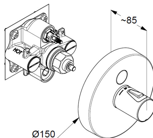
Maßzeichnung
