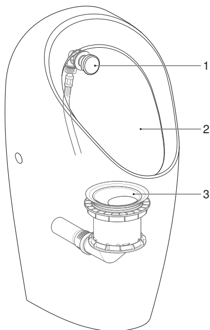
Ilustrimi 1: Pisualet Geberit Selva, Preda dhe Tamina për njësi komandimi inkaso të pisuarit
