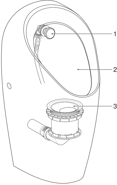
Şekil 1: Ankastre pisuvar deşarj kontrolü için Geberit üreticisine ait Selva, Preda ve Tamina modeli pisuvarlar
