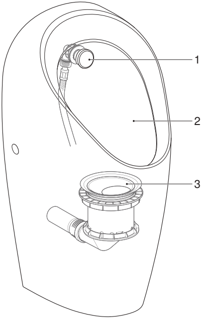
1 الشكل: المبادل Geberit Selva، Preda و Tamina للتحكم في المبادل المثبتة بشكل متساو
