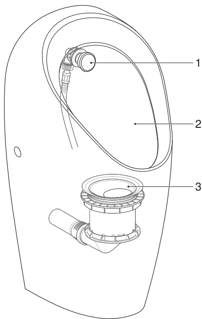
Figura 1: Pisoare Geberit Selva, Preda și Tamina pentru sistemul de comandă a spălării pentru pisoar, încastat
