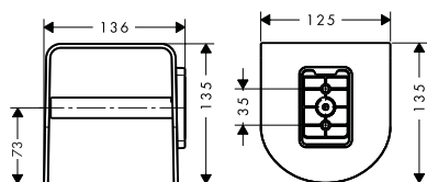
AXOR Urquiola 42436XXX / 42436007
