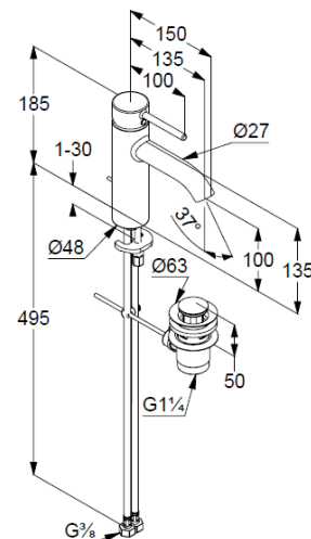
Maßzeichnung/ Dimensional drawing
