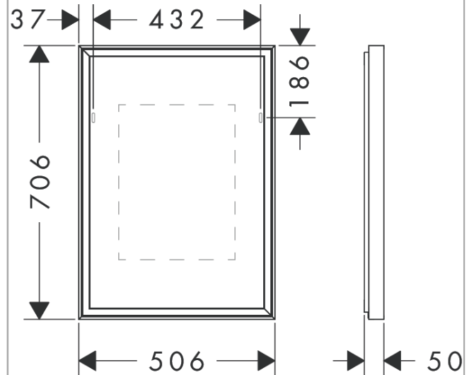
Maßzeichnung
