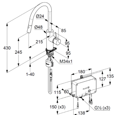
Maßzeichnung/ Dimensional drawing
