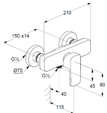
Maßzeichnung/ Dimensional drawing
