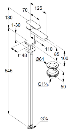
Maßzeichnung/ Dimensional drawing
