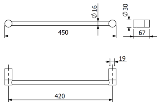
Maßzeichnung/ Dimensional drawing
