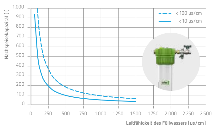
Kapazität der Entsalzung mit Fillsoft I
