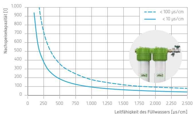
Kapazität der Entsalzung mit Fillsoft II
