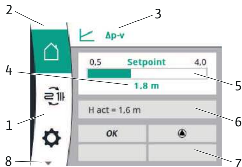
Fig. 7: Schermata principale
