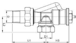
Winkelackergehäuse
