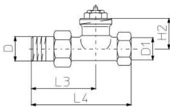
Axialgehäuse
