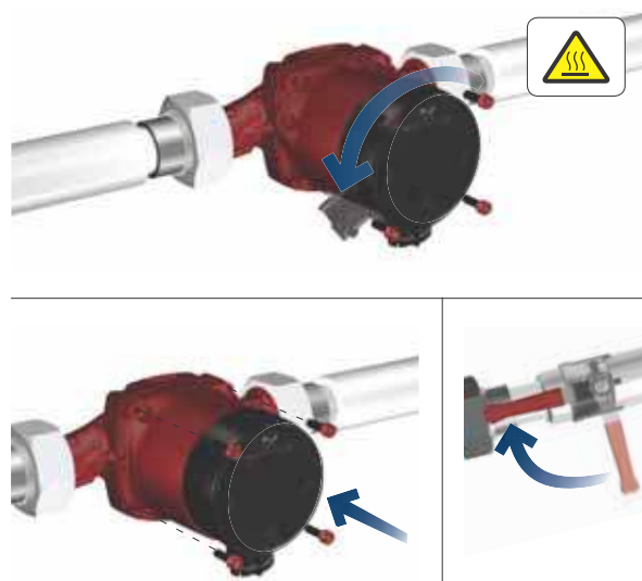
Abb. 3 Positionen des Schaltkastens
