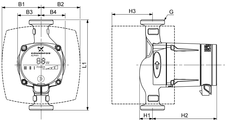
Abb. 17 Maßskizzen, ALPHA1 XX-40, XX-45, XX-60
