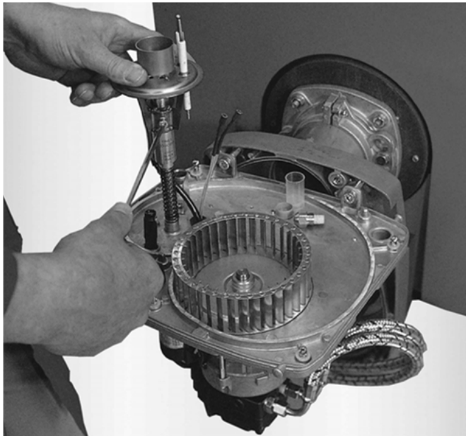
Abb. 37: Demontage Mischsystem
