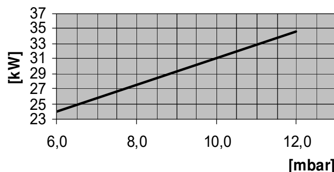
Abb. 21: Leistungsdiagramm RE 1.32 H
