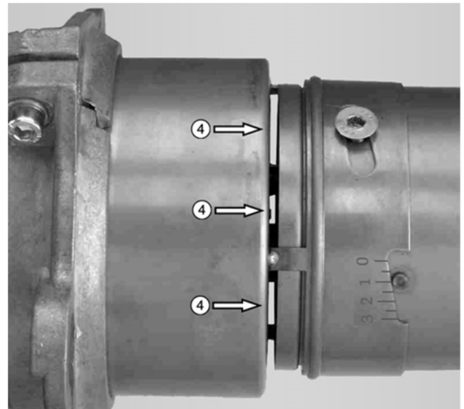
Abb. 9: Rezirkulationsschlitze ④
