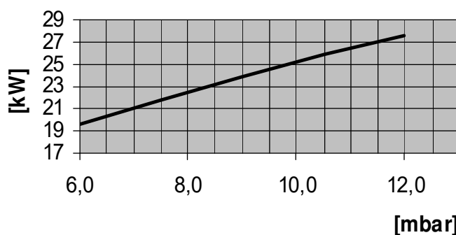
Abb. 20: Leistungsdiagramm RE 1.26 H
