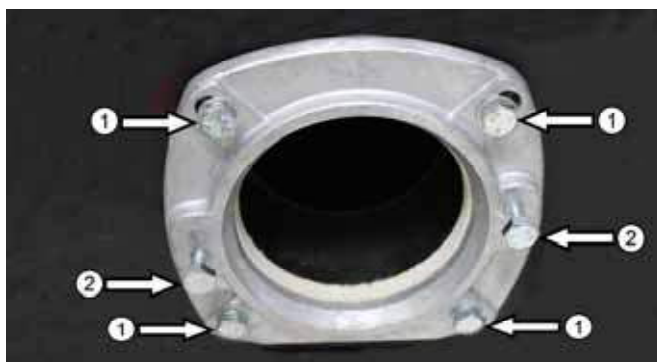
Abb. 6: Befestigung Kesselflansch
