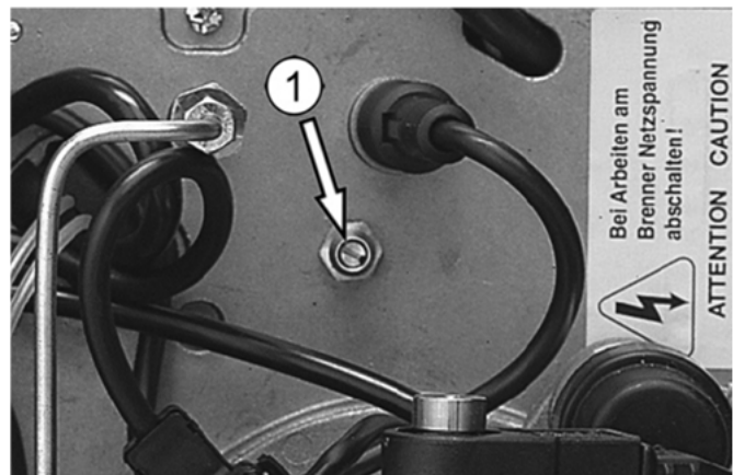
Abb. 27: Messnippel ① zur Prüfung der Gebläsepression
