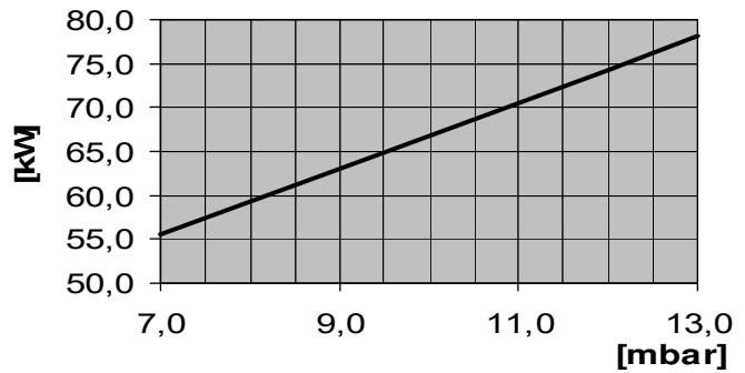
Abb. 26: Leistungsdigramm RE 1.70 H
