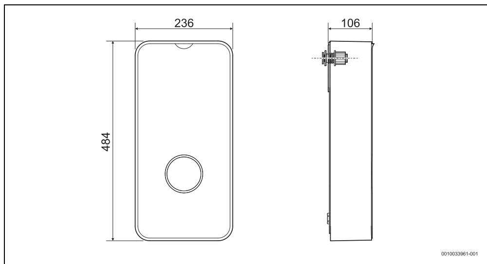
Rys. 54 Wymiary w mm
