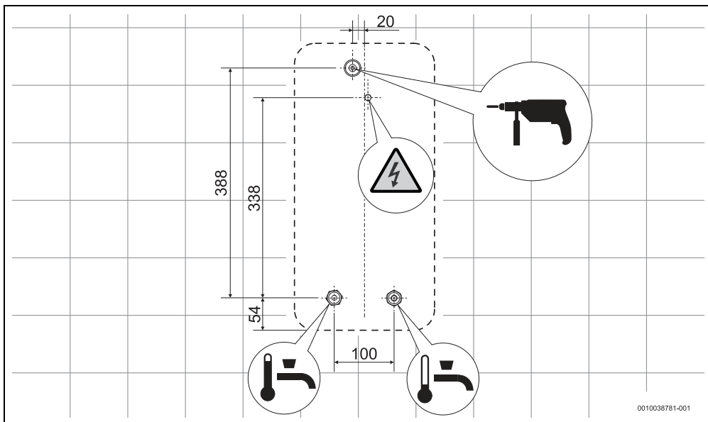
Fig. 30 Dimensions en mm
