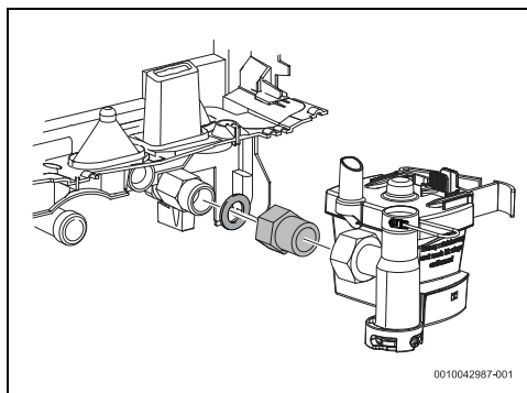
Fig. 45 Bague supplémentaire
