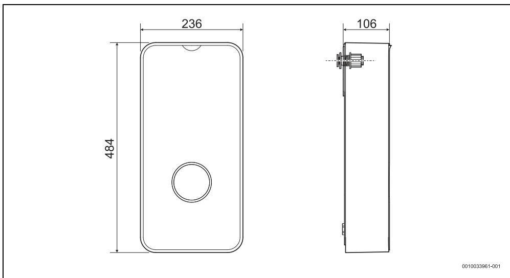
Fig. 29 Dimensions en mm
