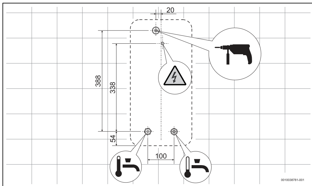
Rys. 55 Wymiary w mm
