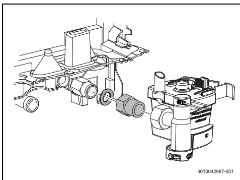
Rys. 70 Dodatkowa tuleja
