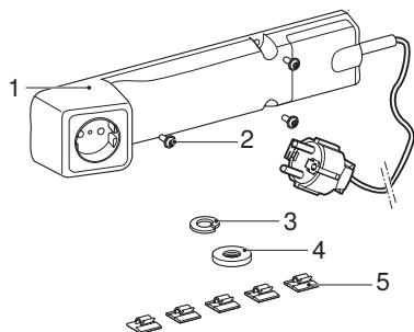
Илустрација 1: Geberit елемент на дозна
