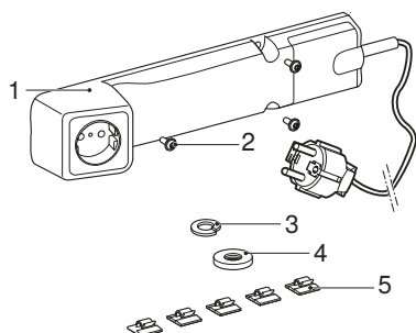
Rysunek 1: Element gniazdka elektrycznego Geberit
