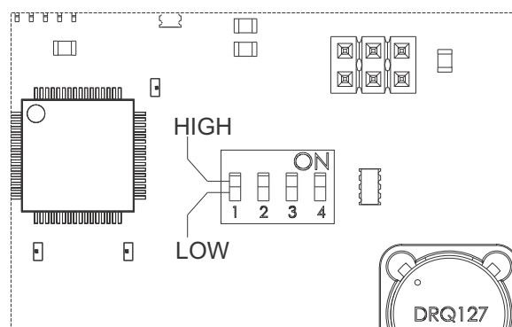
Abb. 16 DIP-Schalter
