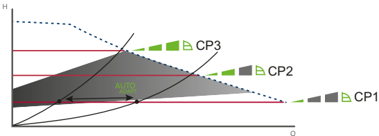
Abb. 26 Drei Konstantdruck-Kennlinien/-Einstellungen
