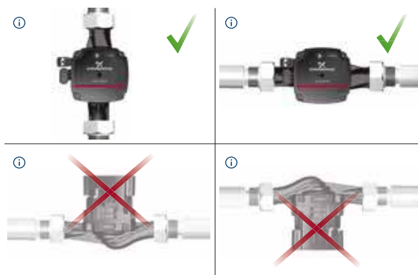
Abb. 7 Position des Schaltkastens, ALPHA SOLAR
