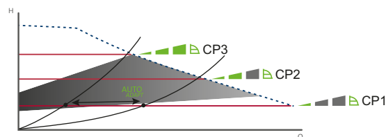
Abb. 24 Drei Konstantdruck-Kennlinien/-Einstellungen
