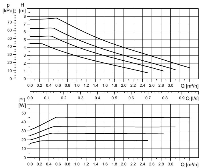
Abb. 51 Leistungskennlinie Hinweis: PBM-Drehzahlkennlinien sind auf Anfrage erhältlich.
