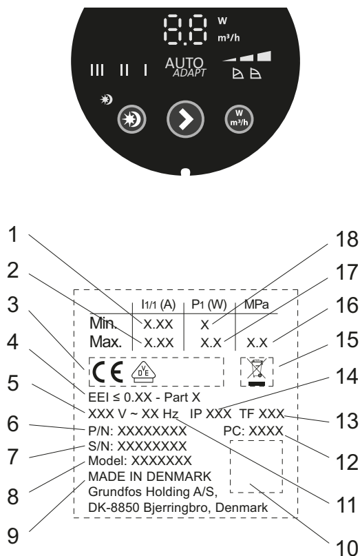
Abb. 18 Typenschild
