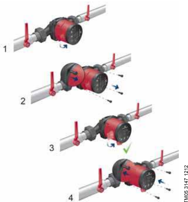
Abb. 5 Verändern der Position des Schaltkastens Der Schaltkasten kann in 90 °-Schritten gedreht werden.
