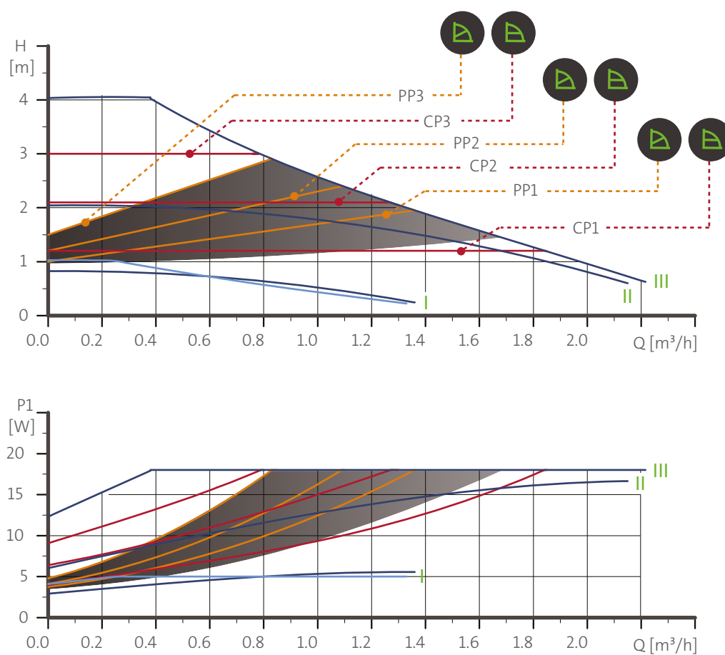
Abb. 40 ALPHA2 und ALPHA3, 25-40 A
