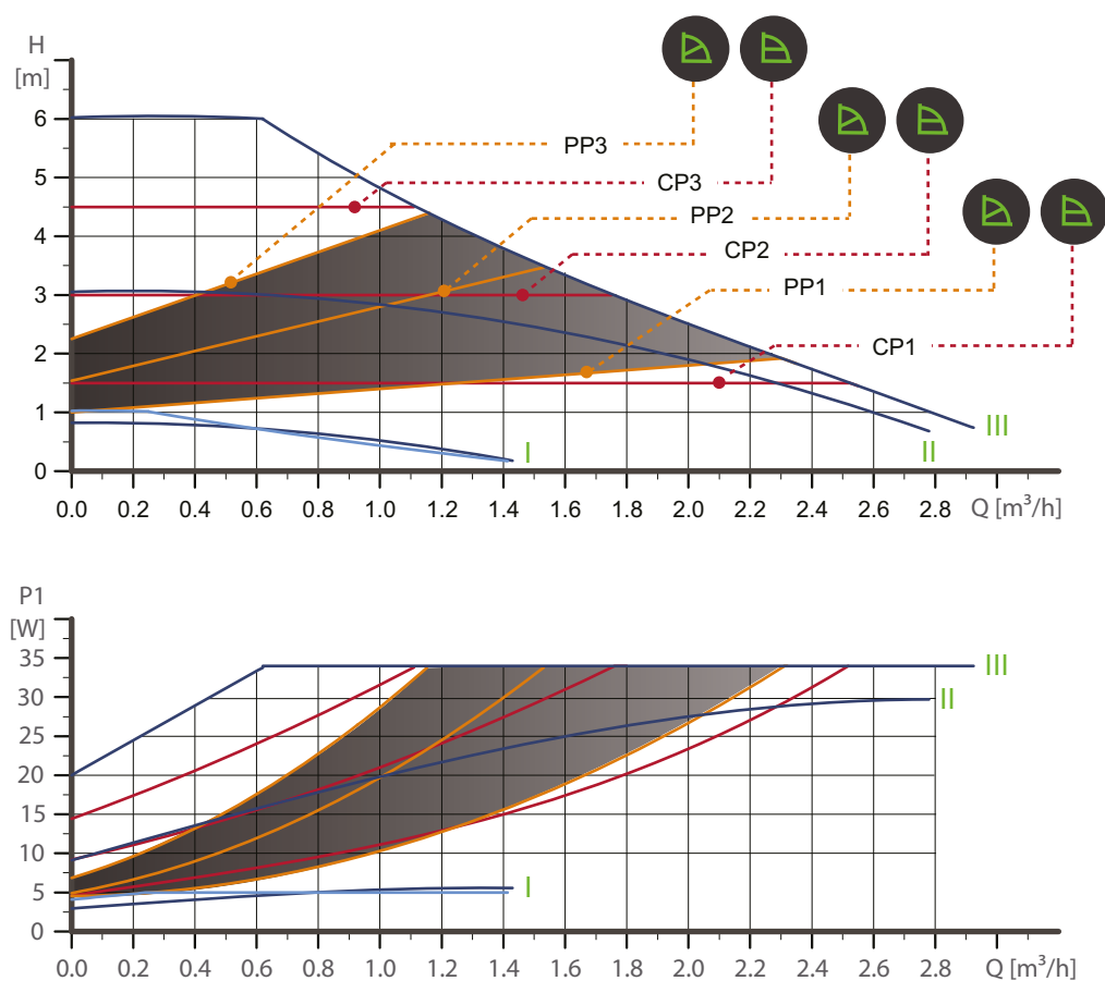
Abb. 41 ALPHA2 und ALPHA3, 25-60 A
