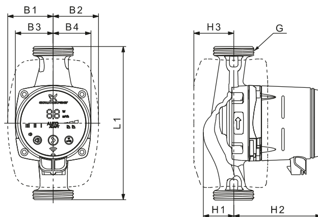
Abb. 34 ALPHA2 und ALPHA3, XX-40, XX-50, XX-60, XX-80
