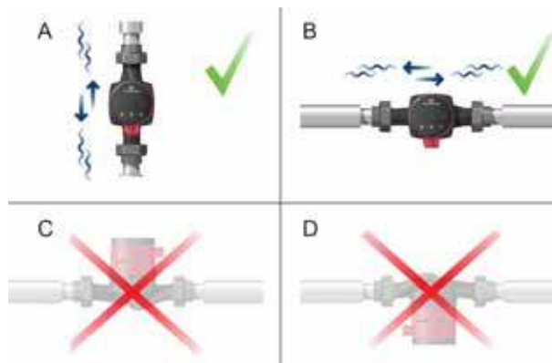
Abb. 2 Position des Schaltkastens
