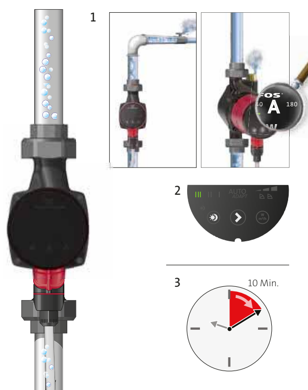
Abb. 14 Entlüften der Heizungsanlage
