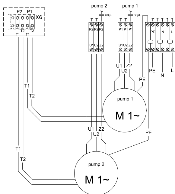
Abb. 27 Schaltplan für einphasige Multilift MD/MLD.12.1.4 und MD/MLD.15.1.4
