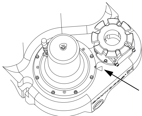
Abb. 34 Ausrichtungsmarkierung am Sammelbehälter und Pumpenflansch
