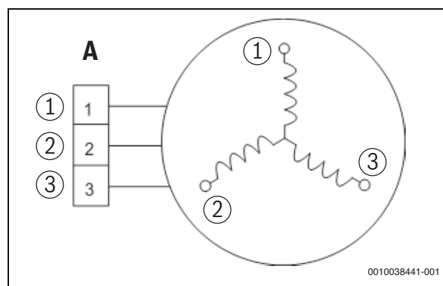
Bild 86 Kompressorprüfung
