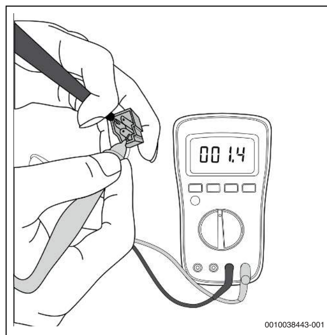
Bild 87 Kompressorprüfung
