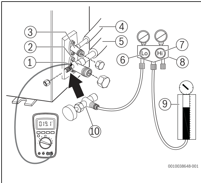
Bild 13 Kältemittelnachfüllung
