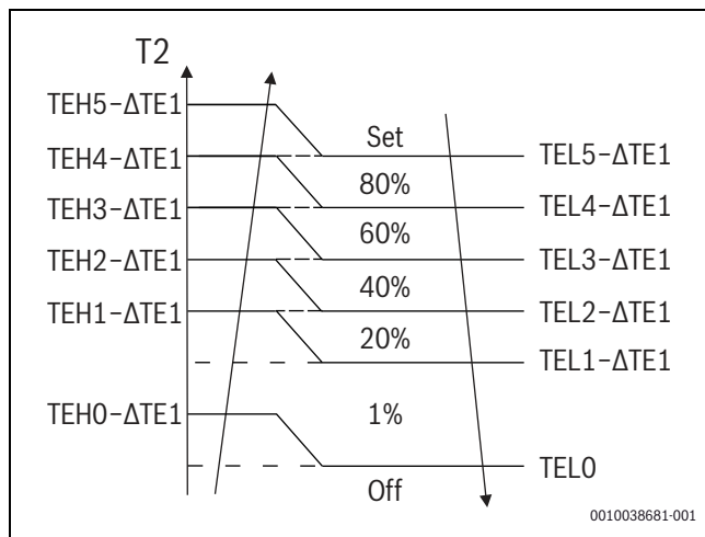
Bild 12 Anti-Kaltluft-Funktion
