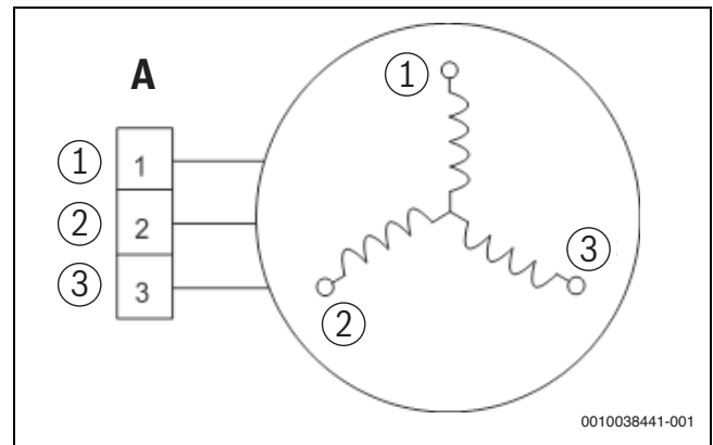
Bild 77 Kompressorprüfung
