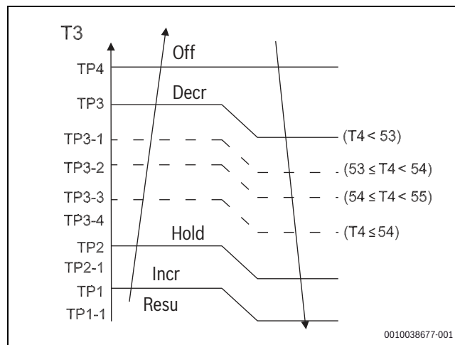
Bild 11 Temperaturschutz für den Verflüssiger
