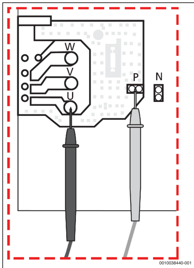
Bild 79 IPM-Durchgangsprüfung
