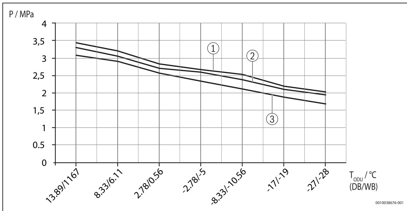
Bild 16 Druck am Wartungsanschluss im Heizbetrieb
