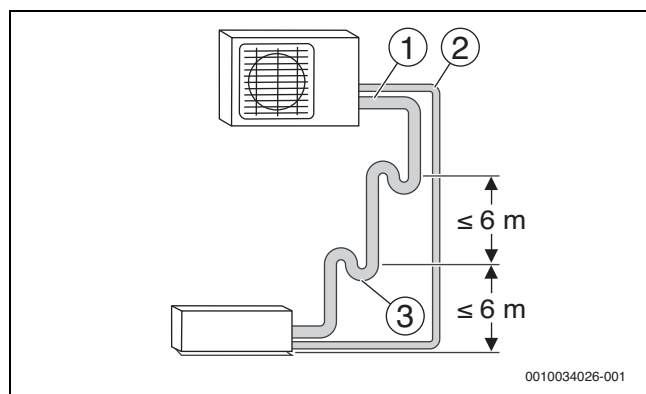
Bild 1 Installation der Außeneinheit über der Inneneinheit
