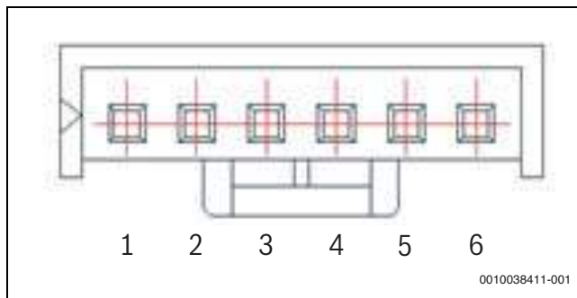
Bild 82 Ventilatormotoranschluss
