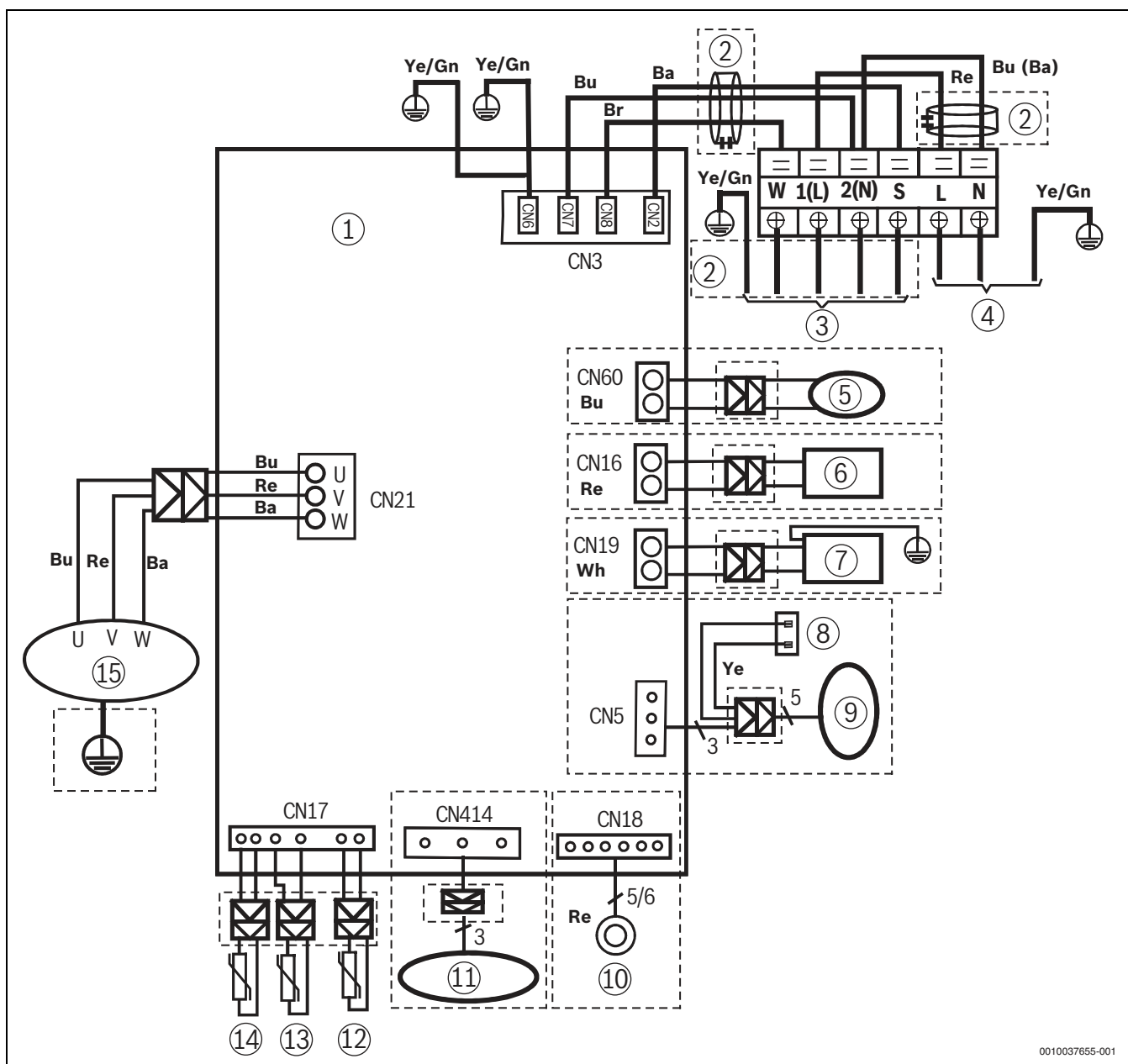
Bild 7 Schaltplan für Außeneinheiten mit 24 kBTU/h
