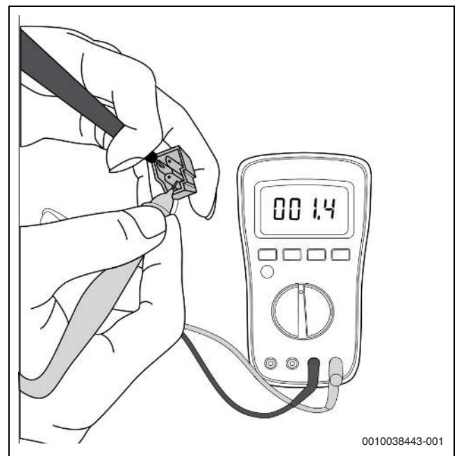
Bild 78 Kompressorprüfung
