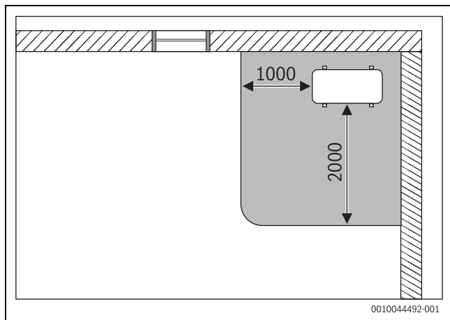
Rys. 3 Strefa ochronna, jednostka zewnętrzna posadowiona na gruncie w narożniku (wymiary w mm)
