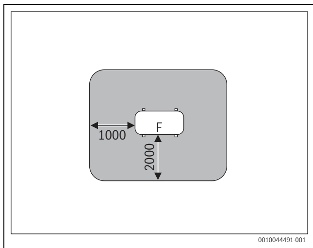
Rys. 2 Strefa ochronna dla urządzenia ustawionego na gruncie na parceli lub na dachu (wymiary w mm)
