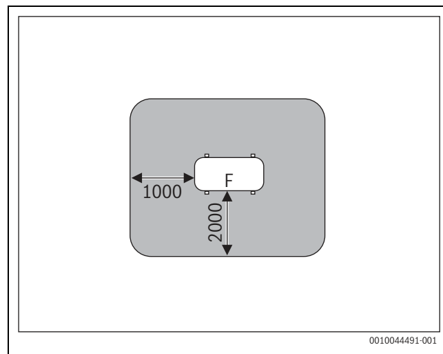
Σχ. 2 Προστατευμένη περιοχή κατά την τοποθέτηση στο δάπεδο στο οικόπεδο ή την οροφή (διάσταση σε mm)
