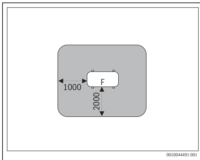
2. ábra Védett terület az ingatlanon a padlón vagy a tetőn felállítva (méretek mm-ben)
