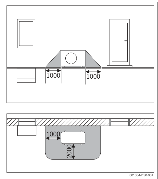
sl. 1 Zona zaštite, stojeća spoljna jedinica na zidu (dimenzije u mm)
