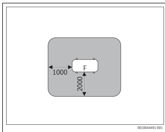
Fig. 2 Sector de protección en caso de instalación sobre el suelo, sobre el terreno o el tejado (medidas en mm)
