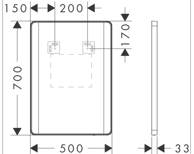
Maßzeichnung
