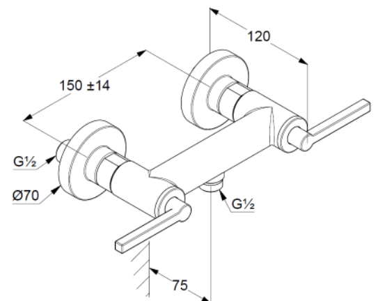
Maßzeichnung/ Dimensional drawing
