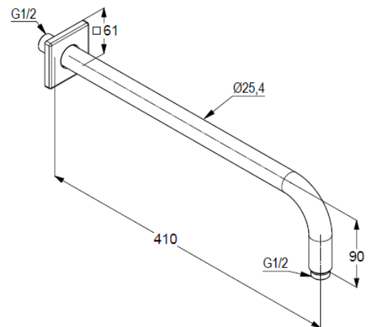
Maßzeichnung/ Dimensional drawing
