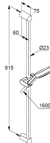
Maßzeichnung/ Dimensional drawing
