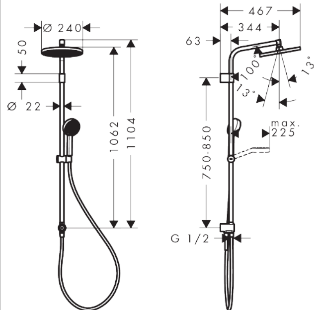
Maßzeichnung
