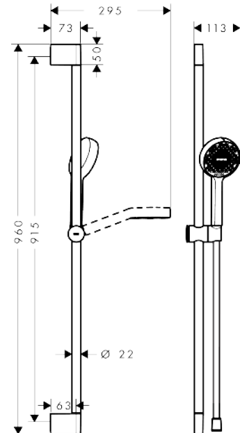
Maßzeichnung
