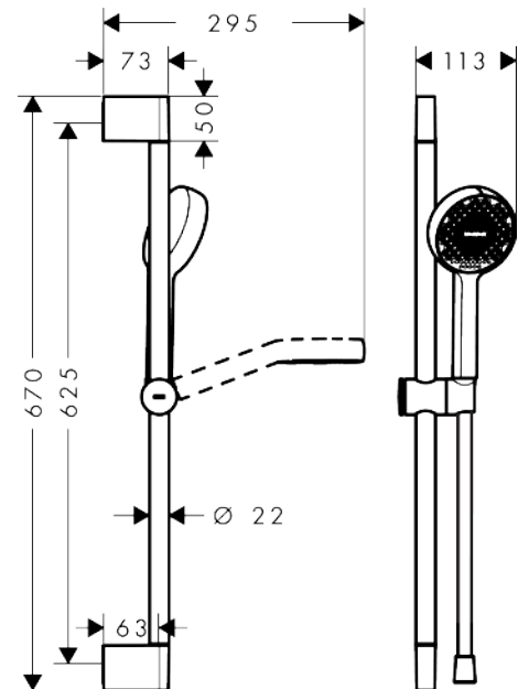
Maßzeichnung
