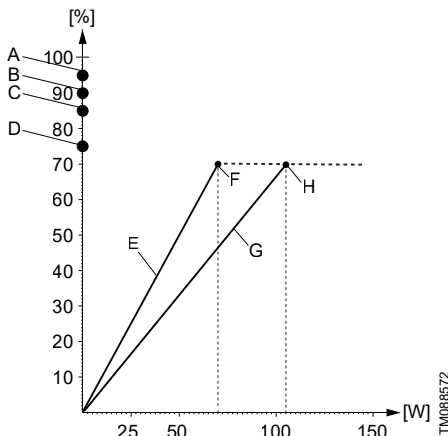
PWM-Rückmeldesignal, Leistungsaufnahme
