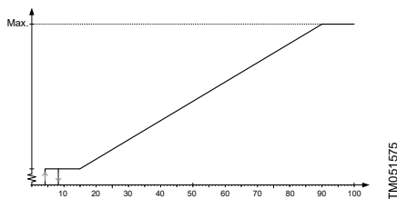
PWM-Eingangssignal C (Solaranlagen)
