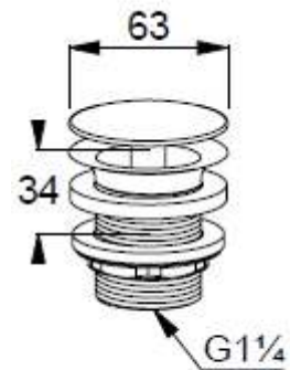
Maßzeichnung/ Dimensional drawing
