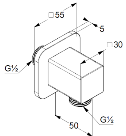
Maßzeichnung/ Dimensional drawing
